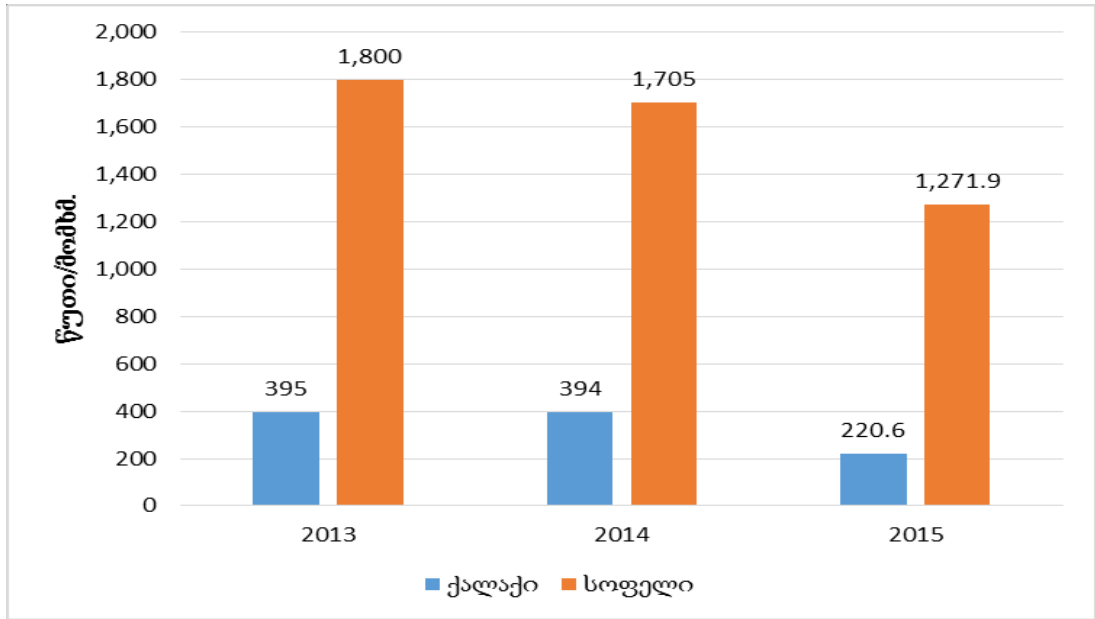
ნახაზი 2.24. სს „კახეთის ენერჯისტირბუციის“ SAIDI-ის მაჩვენებლები 2013-2015 წლებში
