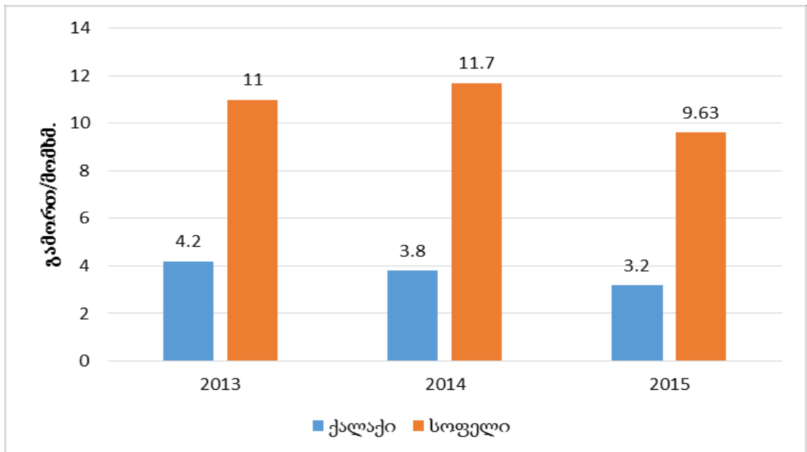
ნახაზი 2.25. სს „კახეთის ენერჯისტირბუციის“ SAIFI-ის მაჩვენებლები 2013-2015 წლებში
